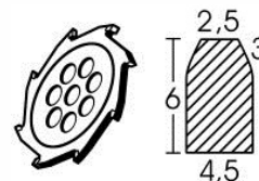
Carbide blade Ø 110 x 4.5 mm
