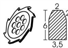
Carbide blade Ø 110 x 3.5 mm
